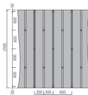
Anwendung Ständerwerk 300 mm mit Dämmplattentellern und Schrauben für BA 10; BA 12,5 mm.
