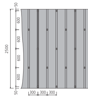
Anwendung Ständerwerk 300 mm mit Dämmplattentellern und Schrauben für BA12,5 mm.
